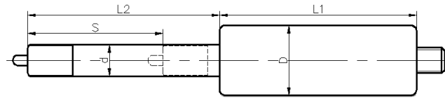
L1-缸筒长度 L2-活塞杆伸出长度 D-缸筒直径 d-活塞杆直径 S-行程
